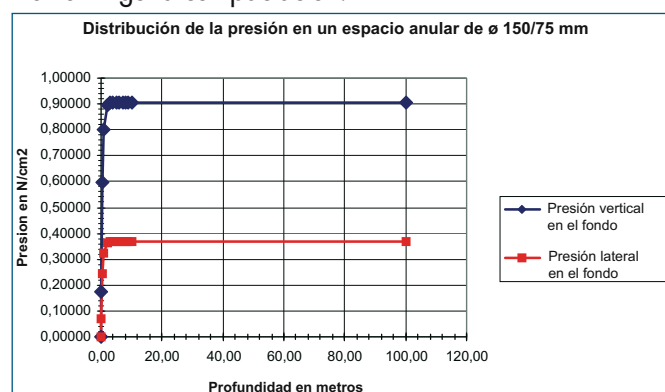
Diagrama 1: Distribución de la carga en el espacio anular del sondeo relleno de grava Ø perforación 150 mm / Ø tubo rígido roscado NORIP DN 65
